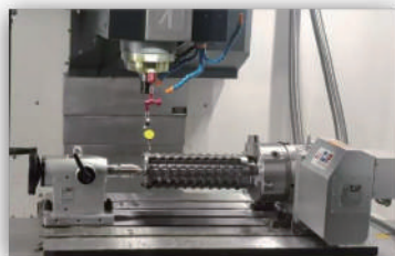
▲ RC-210 + TTJ-210
