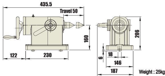
TTJ-210/255
