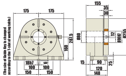
Weight : 57kg
